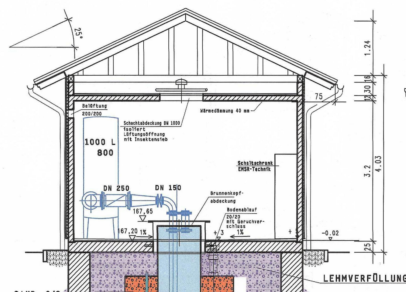
Schnitt B - B
