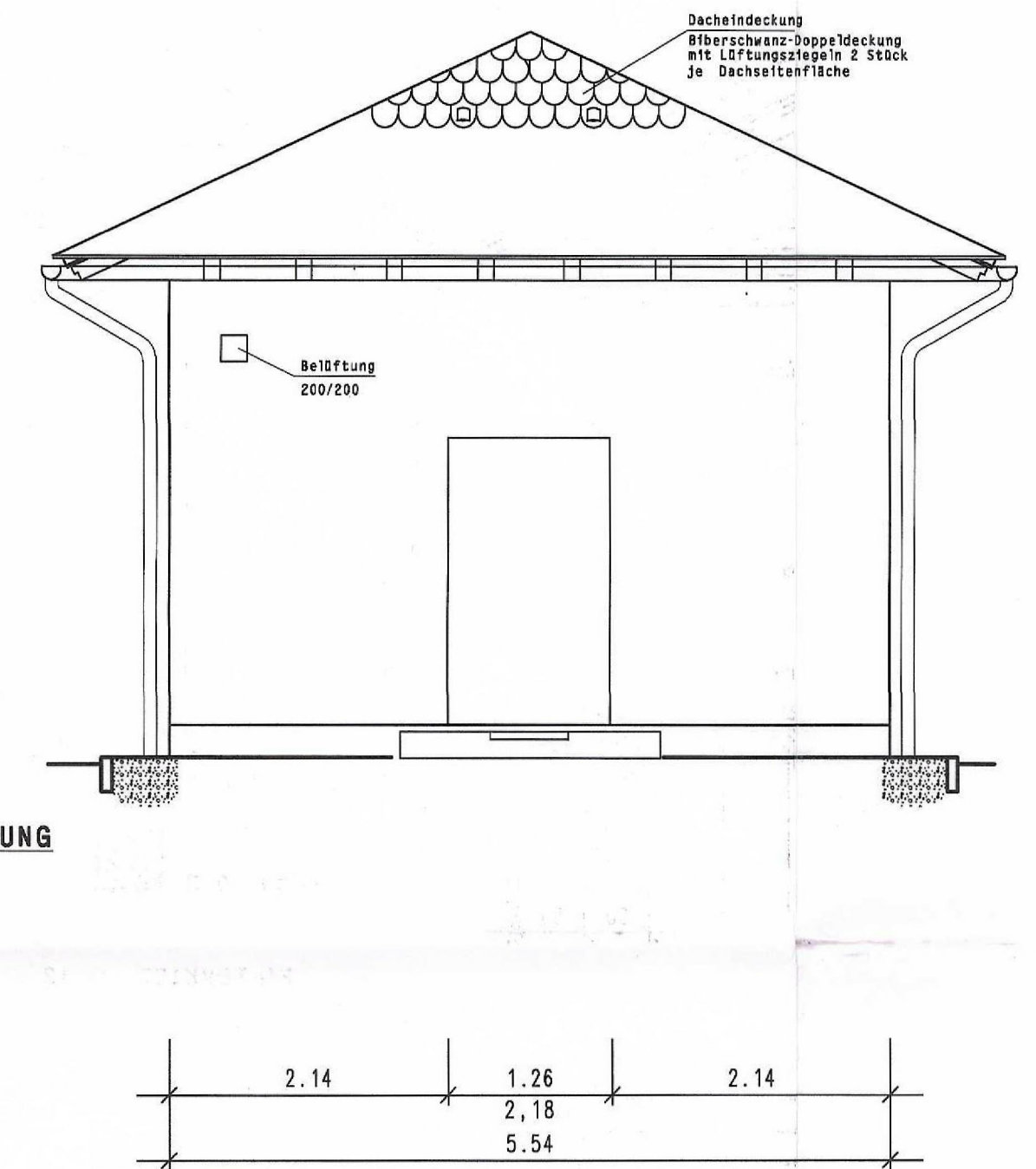
Ansicht Süd - West
