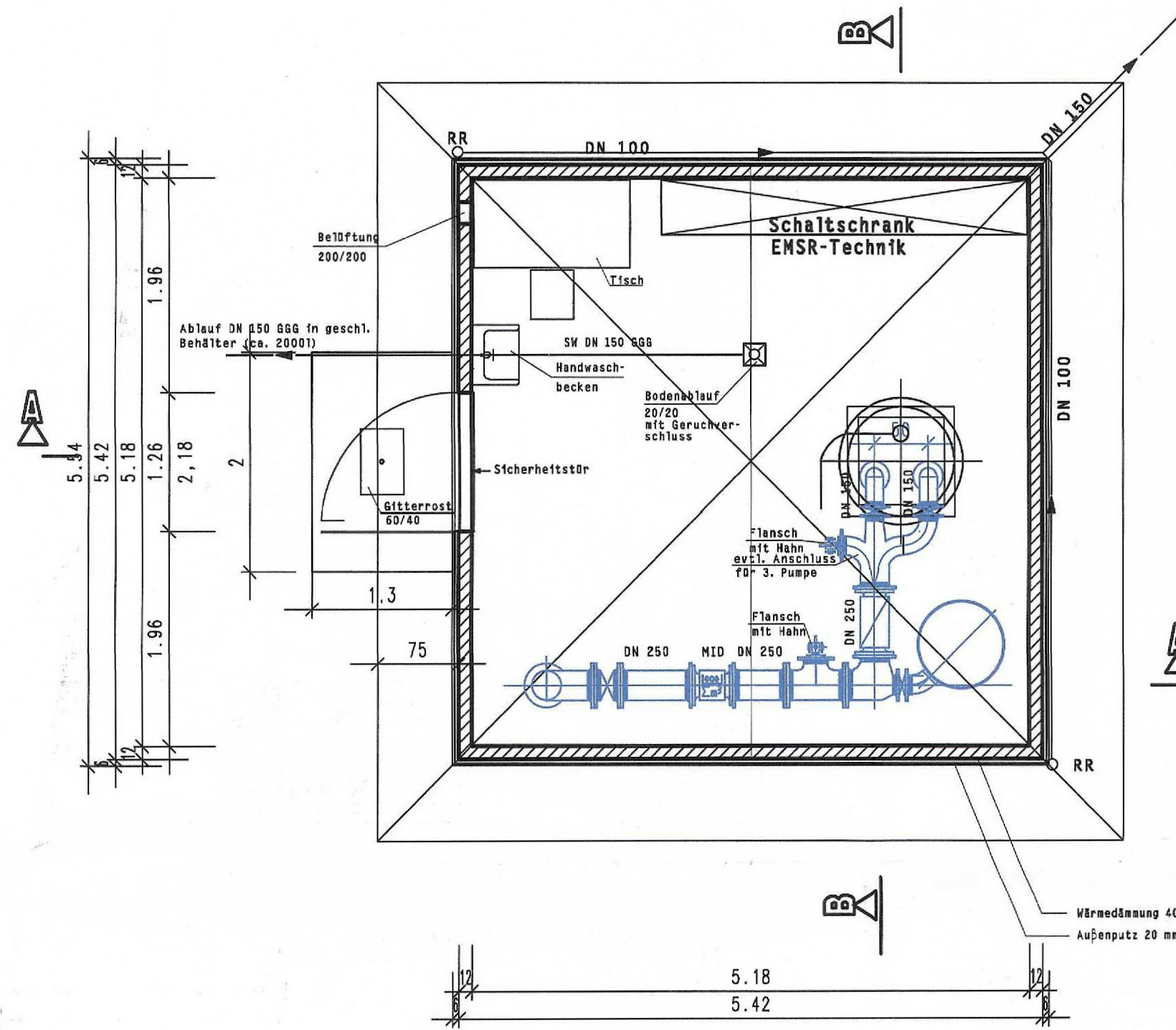
Grundriss
