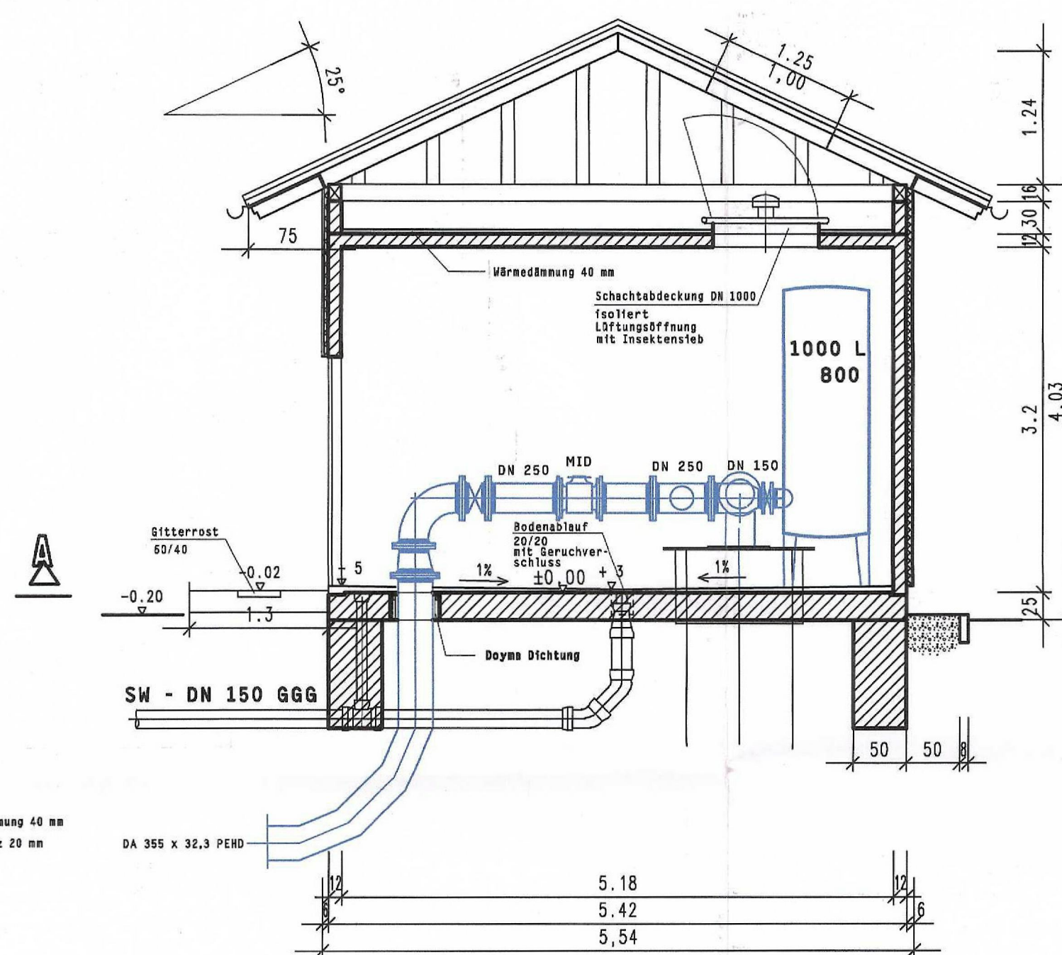
Schnitt A - A
